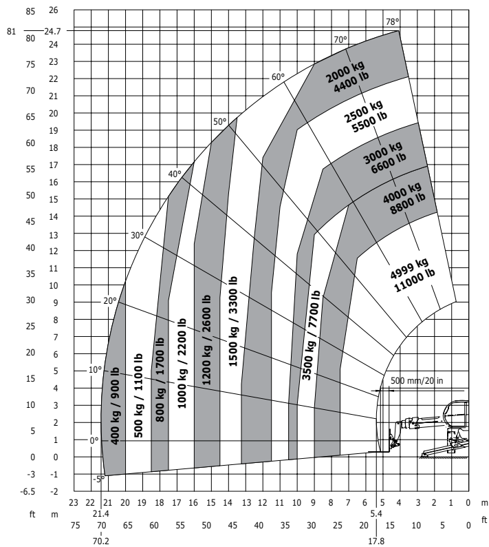
Drehung auf ausgefahrenen Stützen mit Gabelzinken
